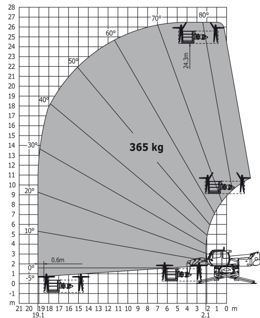
Rotatie op verlaagde stabilisatoren met 1500 kg giek
